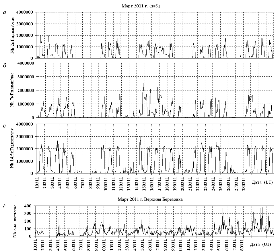
Рис. 3. Суточные вариации аддитивной смеси естественного и антропогенного электромагнитного излучения на частотах 2; 7; 14,5 кГц (здание ИФМ СО РАН) (а–в); суточный ход ЕИЭМПЗ на частоте 14,5 кГц (Верхняя Березовка) (г)
