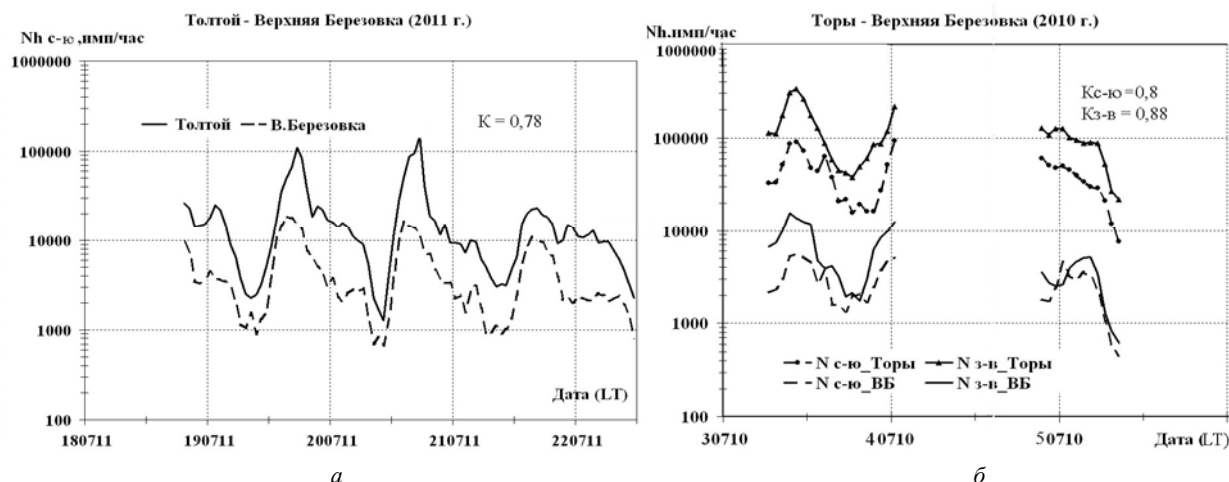
Рис. 1. Результаты регистрации магнитной составляющей ОНЧ-импульсного потока на частоте 14,5 кГц в пунктах наблюдения:
