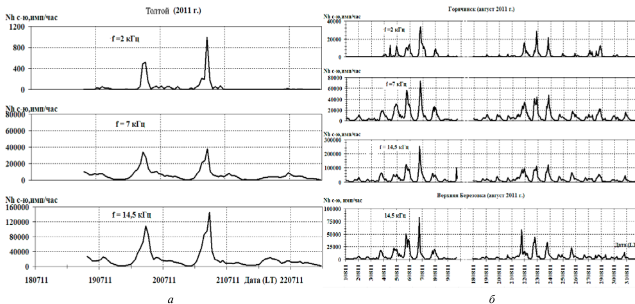
Рис. 2. Результаты регистрации магнитной составляющей ОНЧ-импульсного потока на частотах 2, 7 и 14,5 кГц: а – в ПН «Толтой» 18–22 июля 2011 г.; б – в ПН «Горячинск» и «Верхняя Березовка» в августе 2011 г.
