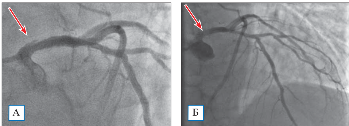
Рис. 3. Тот же пациент: селективная коронарография левой коронарной артерии.
