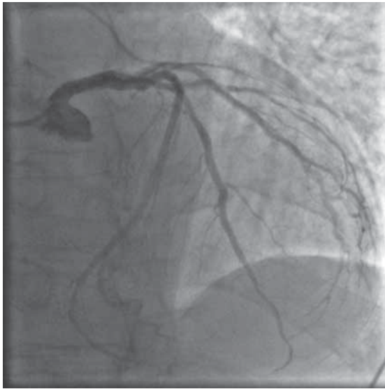
Рис. 5. Тот же пациент: результат стентирования ствола левой коронарной артерии.
