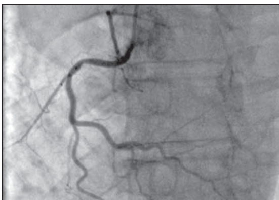
Рис. 4. Тот же пациент: селективная коронарография правой коронарной артерии.
