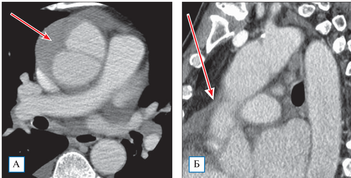
Рис. 2. Тот же пациент: КТ-аортография.
