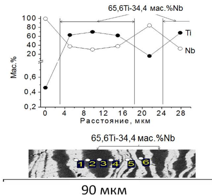
Рис. 5. К результатам локального РСА: концентрационные профили титана и ниобия и фрагмент микроструктуры Nb/Ti-композита 13\text{NbTi}_2 после ДС и ПП 1-го цикла
