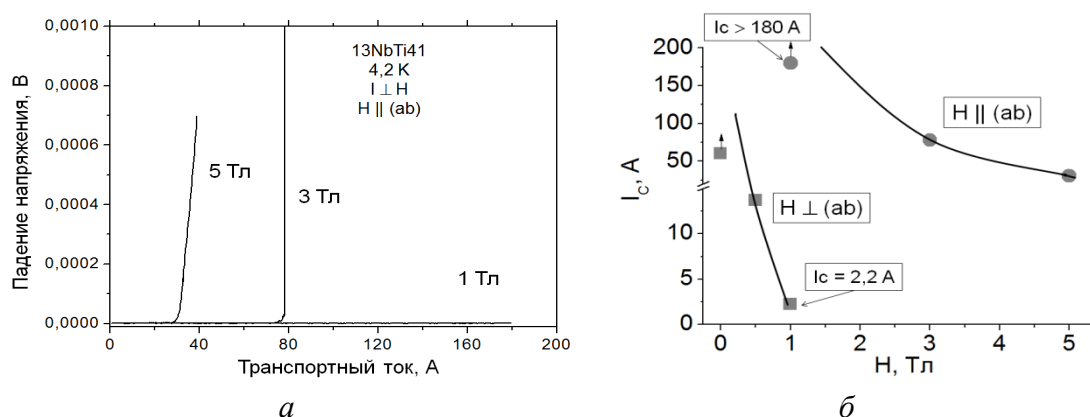
Рис. 10. Вольт-амперные характеристики многослойной сверхпроводящей ленты из сплава Nb–Ti при H \parallel (ab) и H = 1, 2 и 3 Тл (а) и зависимости I_c(H) при H \parallel (ab) и H \perp (ab) (б)
