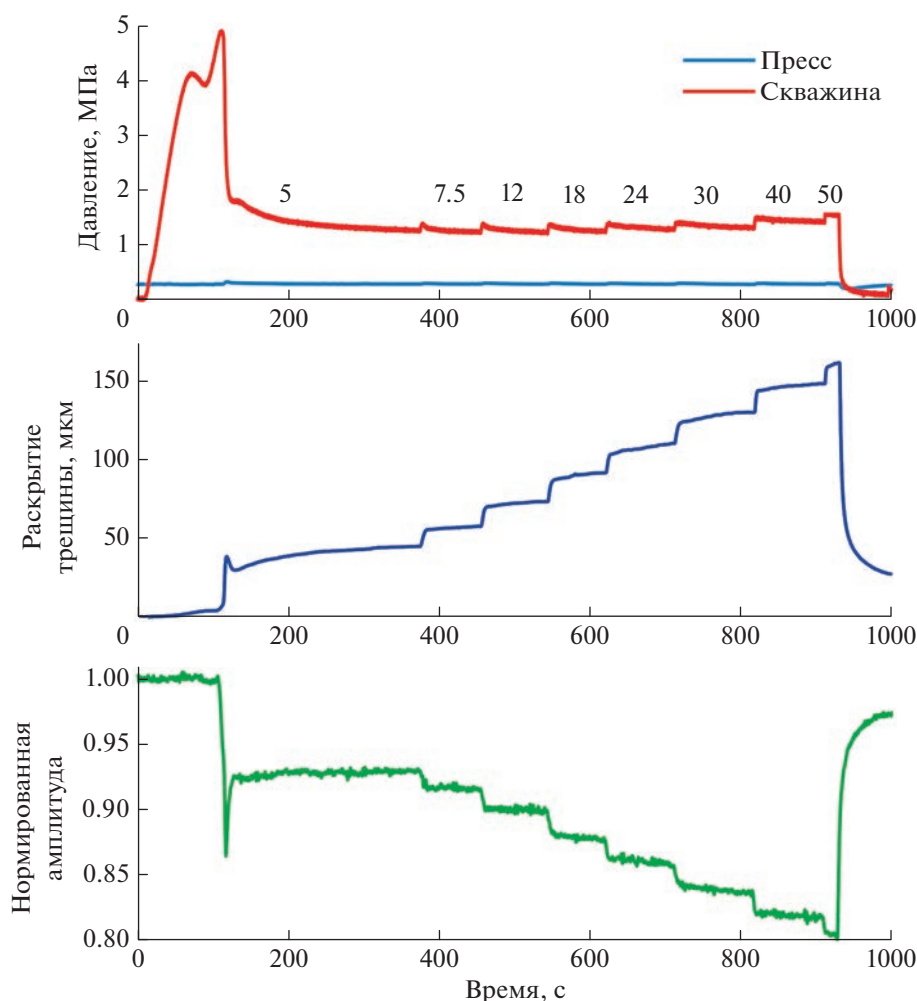
Рис. 3. Синхронизированные по времени записи давления в рабочей скважине, гидравлическом прессе, создающем вертикальное давление, с величиной раскрытия трещины гидроразрыва и с амплитудой прошедшего ультразвукового импульса, нормированной на его амплитуду до возникновения трещины гидроразрыва. Числа над последовательными участками кривой давления в скважине показывают величину расхода рабочей жидкости на каждой ступени увеличения расхода в \text{см}^3/\text{мин} .
