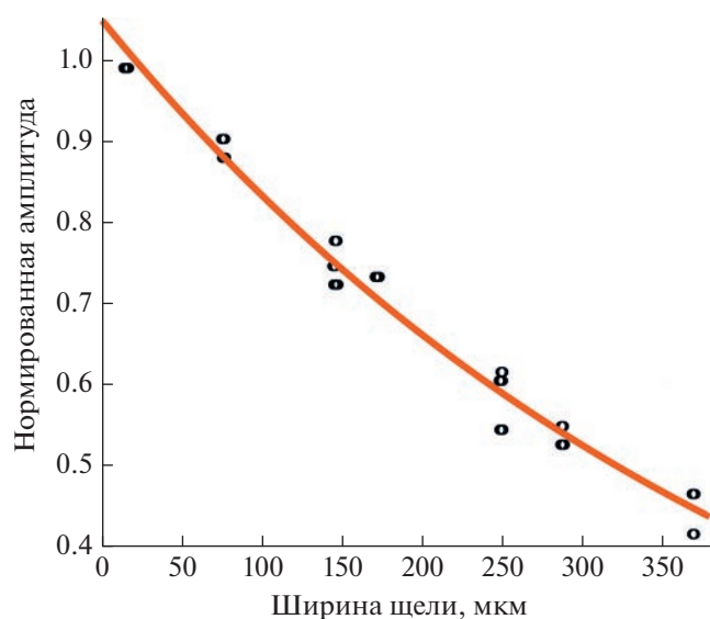
Рис. 5. Зависимость амплитуды ультразвукового импульса, прошедшего через щель между стеклянными пластинами от ее ширины.
