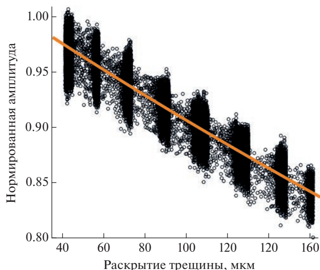
Рис. 4. Зависимость амплитуды ультразвукового импульса, прошедшего через трещину гидроразрыва от величины ее раскрытия в эксперименте с образованием трещины гидроразрыва в исходном образце. Амплитуда нормирована на ее значение при раскрытии, равном 20 мкм.
