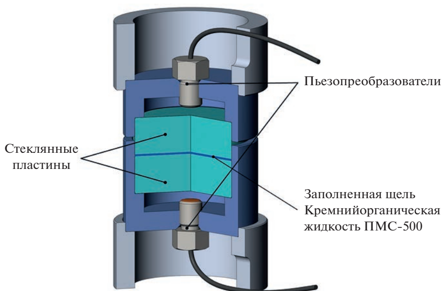
Рис. 2. Схема сборки для исследования прохождения ультразвука через щель между стеклянными пластинами.
