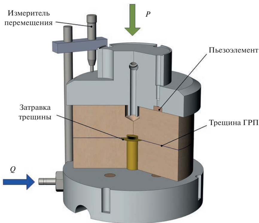
Рис. 1. Схема экспериментальной сборки для исследования прохождения ультразвука через трещину гидроразрыва. Чтобы не загромождать рисунок, показана только одна стойка с измерителем перемещения.
