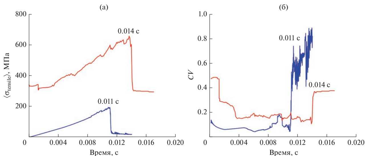
Рис. 5. Усредненные по слоям максимальные растягивающие напряжения (а) и их коэффициенты вариации (б): синие кривые — однородный образец, красные кривые — гетерогенный образец. Метки времени позволяют сопоставить характерные точки изменения напряжений и их коэффициентов вариации.
