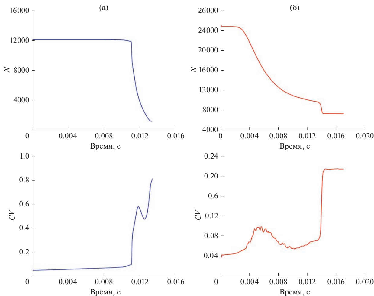
Рис. 4. Зависимости от времени числа целых связей усредненных по слоям ( N ) и коэффициента вариации ( CV ): (а) – однородный образец; (б) – гетерогенный образец.
