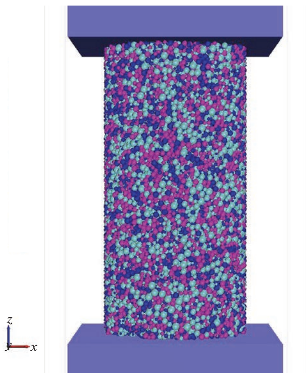
Рис. 1. Образец и схема модельного эксперимента. Пример гетерогенного образца: частицы из разного материала окрашены в разный цвет. Плиты моделируют пуансоны прессы.
