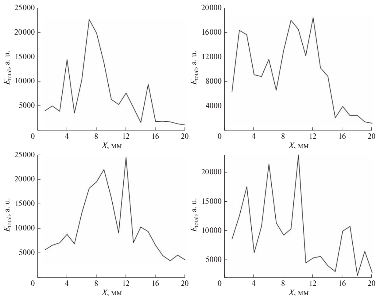
Рис. 8. Изменение суммарной энергии сигналов АЕ по координате (высоте образца) при деформировании образца гранита Westerly.
