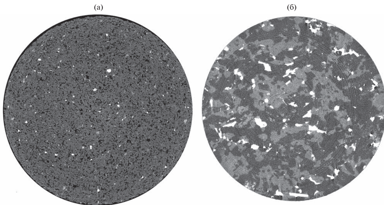
Рис. 6. Примеры томографических срезов: (а) — песчаник Berea; (б) — гранит Westerly. Градации серого соответствуют различной плотности материала: наиболее плотным фракциям соответствует белый цвет, пустотам (поры, трещины и т.д.) — черный цвет.
