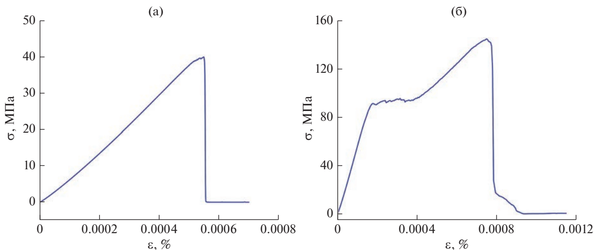
Рис. 2. Диаграммы нагружения (напряжение ( \sigma ) — деформация ( \varepsilon )) при деформировании однородного (а) и гетерогенного (б) образцов.
