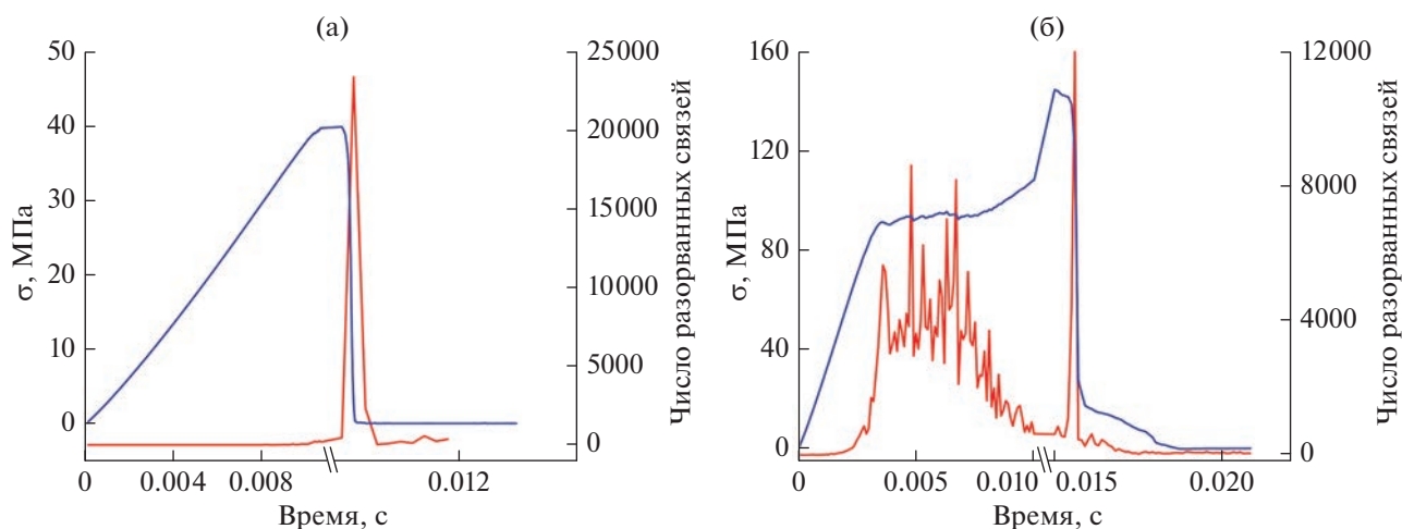
Рис. 3. Изменение напряжения (синие кривые) и активность акустической эмиссии (красные кривые) при деформировании однородного (а) и гетерогенного (б) образцов.
