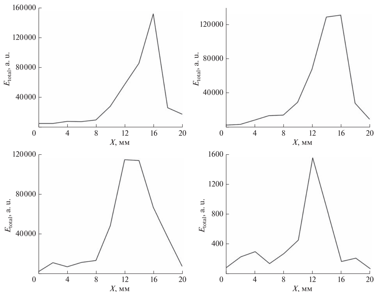
Рис. 7. Изменение суммарной энергии сигналов АЕ по координате (высоте образца) при деформировании образца песчаника Berea.
