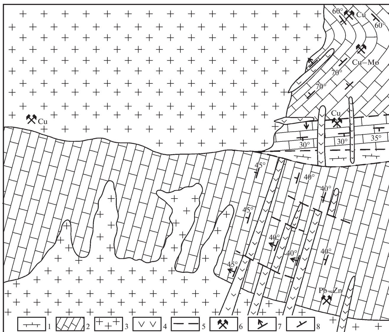
Фиг. 6. Схематический план размещения структур месторождения Юлия, по В.М. Крейтеру (1956) с небольшими изменениями. 1 – массивные известняки ( Cm_1 ); 2 – тонкослоистые известняки ( Cm_1 ); 3 – интрузивы сиенитов, кварцевых сиенитов и кварцевых монцонитов; 4 – дайки преимущественно монцодиорит-порфиров; 5 – разломы; 6 – пункты оруденения медного (с Mo, Au) и Pb-Zn; 7, 8 – элементы залегания: 7 – контактов, 8 – слоистости.
