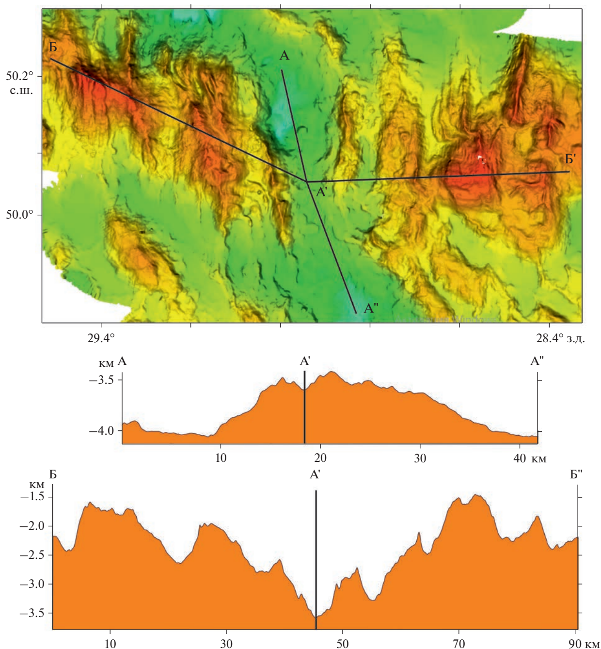
Рис. 7. Рельеф океанского дна и профили в районе ТМС-3.
