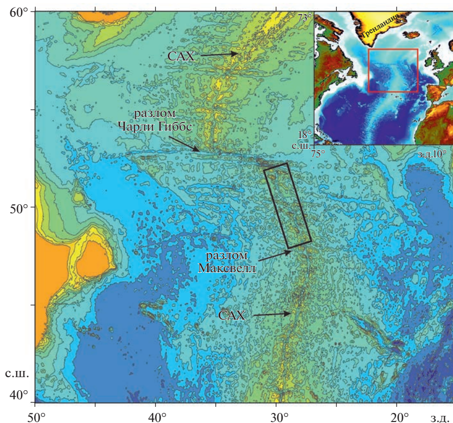
Рис. 1. Карта рельефа дна Северной Атлантики.
