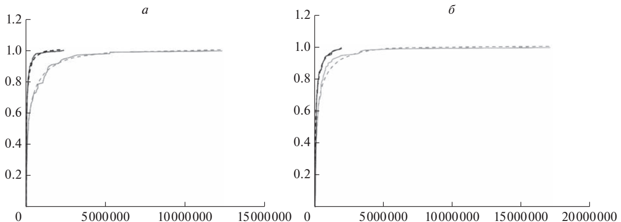
Рис. 5. Примеры графиков распределения площадей термокарстовых озер на участках 22 (а) и 28 (б): по оси x даны площади озер ( \text{м}^2 ), по оси y — вероятность; черные линии — графики озер, возникших на поверхности массивов хасыреев, серые — на основной поверхности; сплошные линии — эмпирические распределения площадей, штриховые — теоретические интегрально-экспоненциальные.
