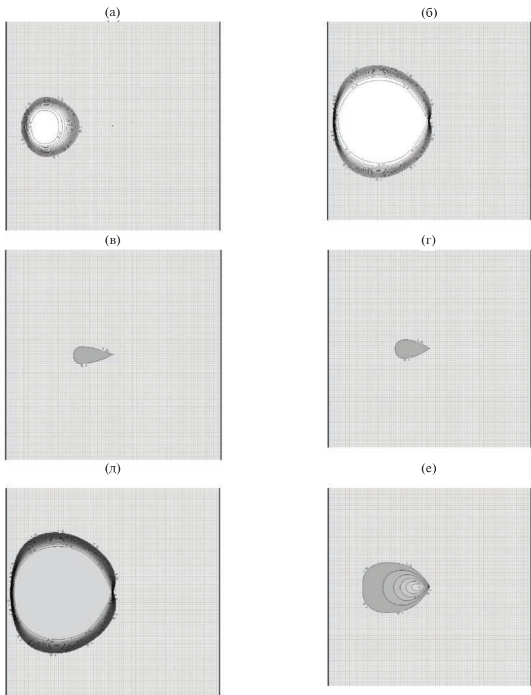
Рис. 10. Положение линзы распресненных вод на следующие моменты времени от начала эксплуатации инфильтрационного бассейна системы ИППВ: а – 20 сут (начало пролива), б – 90 сут (конец пролива), в – 365 сут (конец 1 года), г – 2165 сут (конец 6-го года, 1-й год без ИППВ), д – 5550 сут (15-й год, после ИППВ), е – 5770 сут (конец 15-го года).
