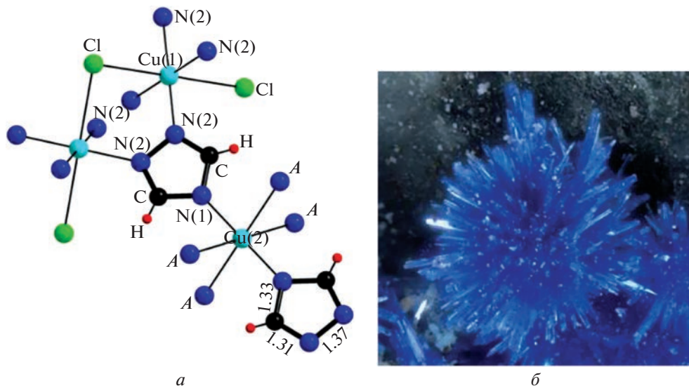
Рис. 4. Основной фрагмент структуры чанабаяита, объясняющий связь между полиэдрами \text{Cu}^{2+} катионов. А-позиции заняты замещающими друг друга различными компонентами [ A = (\text{NH}_3)_{0.50}(\text{H}_2\text{O})_{0.125}(\text{OH})_{0.075}\text{Cl}_{0.175} ] (а) (Чуканов и др., 2015). Кристаллы чанабаяита темно-синего цвета (б).
