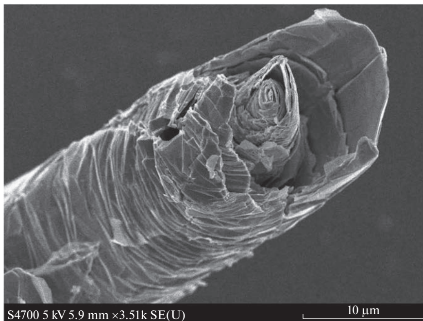
Рис. 11. Свернутые в трубки слоистые модули в структуре мереланиита. Снимок получен на сканирующем электронном микроскопе высокого разрешения Hitachi s 4700 (Jaszczak et al., 2016).
