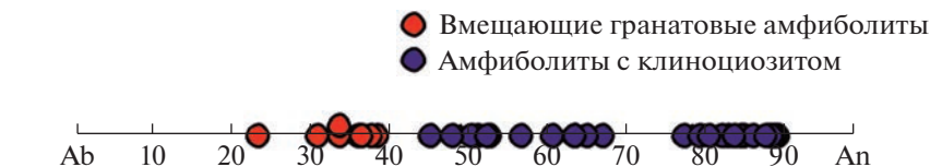
Рис. 5. Диаграмма составов плагиоклаза из клиноцизитовых и вмещающих гранатовых амфиболитов.
