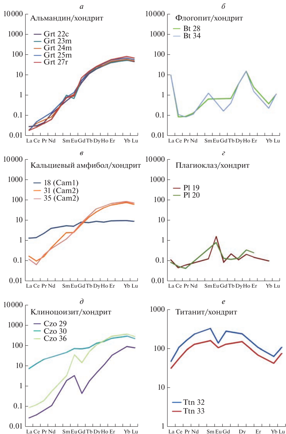
Рис. 7. Спектры распределения REE в минералах из клиноцоизитовых амфиболитов.
